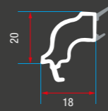
ER 6008 Dekoratif Çift Cam Çıtası ER 6008 Dec. Double Glazing Bead
