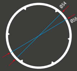
ER 6011 Boru Profili ER 6011 Pipe Profile
